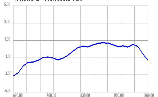
690.00MHz - 960.00MHz Gain
