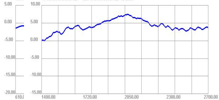
611 1400.00MHz - 2700.00MHz Gain
