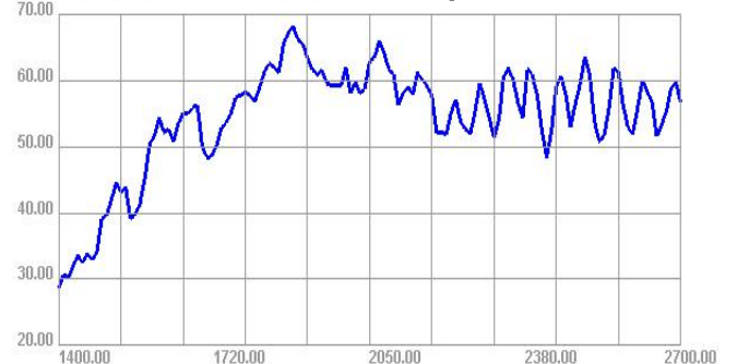
1400.00MHz - 2700.00MHz Efficiency
