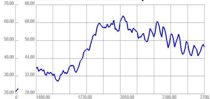
6 1400.00MHz - 2700.00MHz Efficiency
