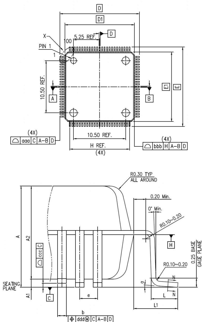
图21 LQFP100 封装图
